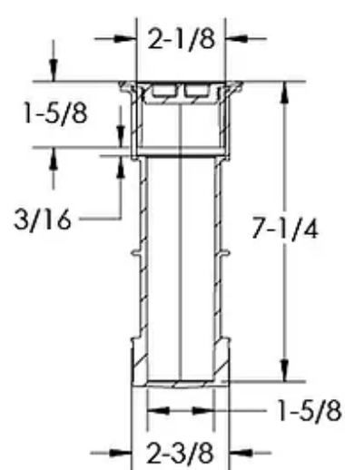
SECTION A-A
